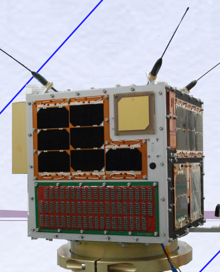
HORYU-IV
